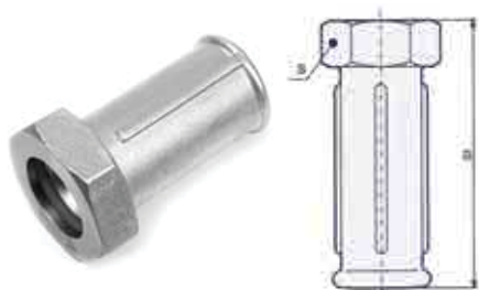
GH SPOJKA
