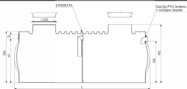
2 - prekatna greznica
