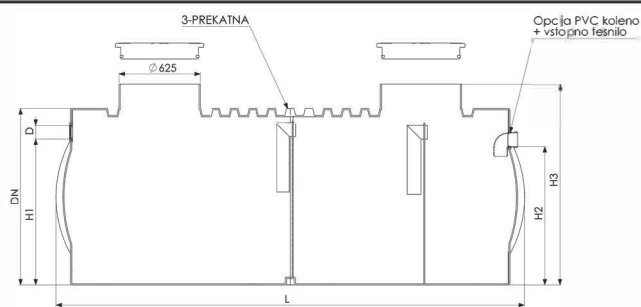
3 - prekatna greznica
